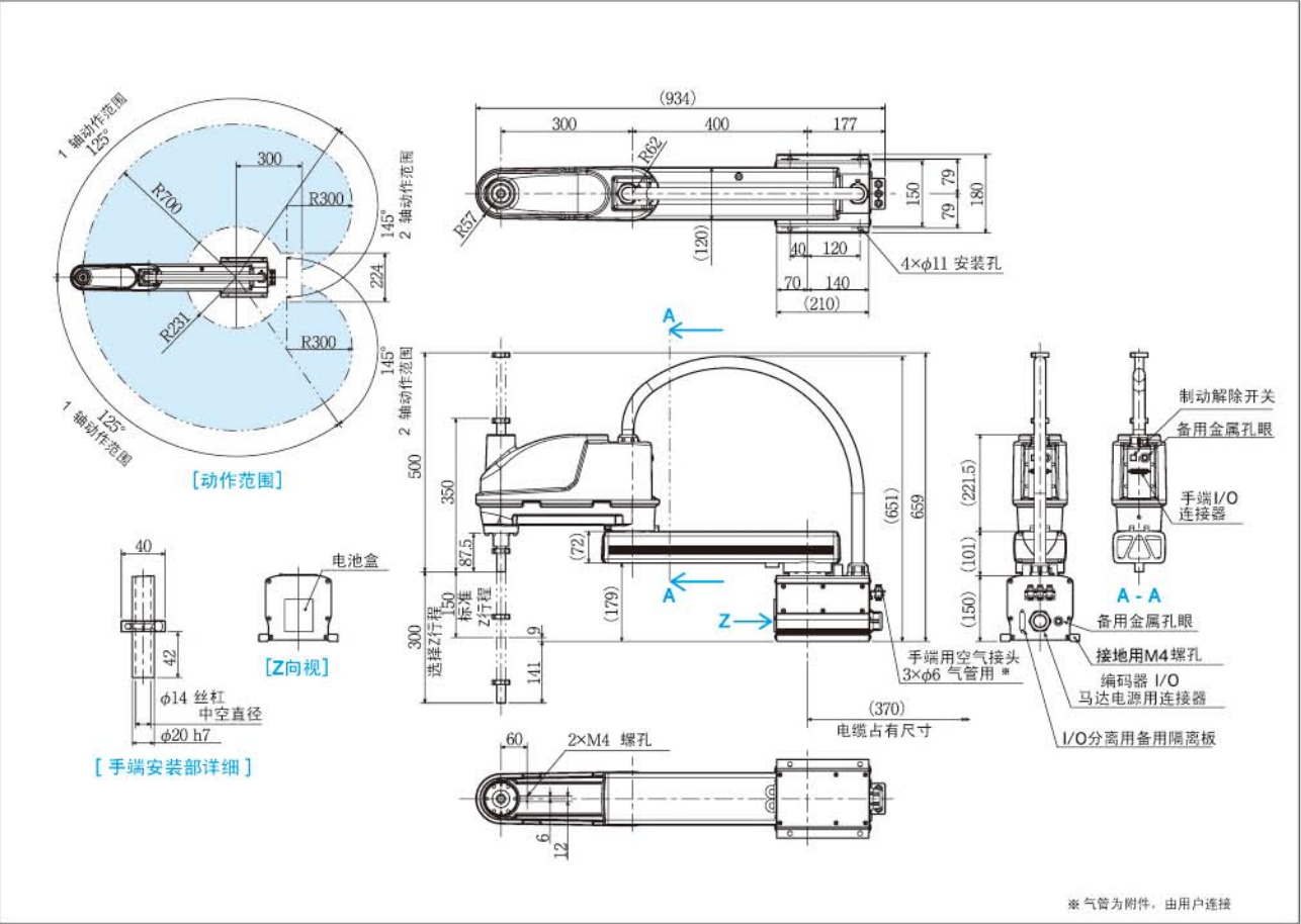
THL700外形图
