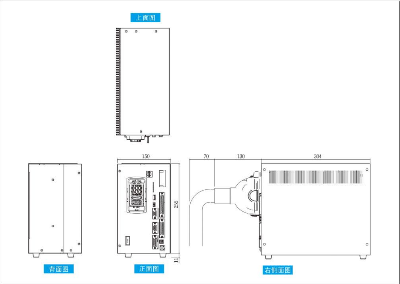
TSL3000外形图
